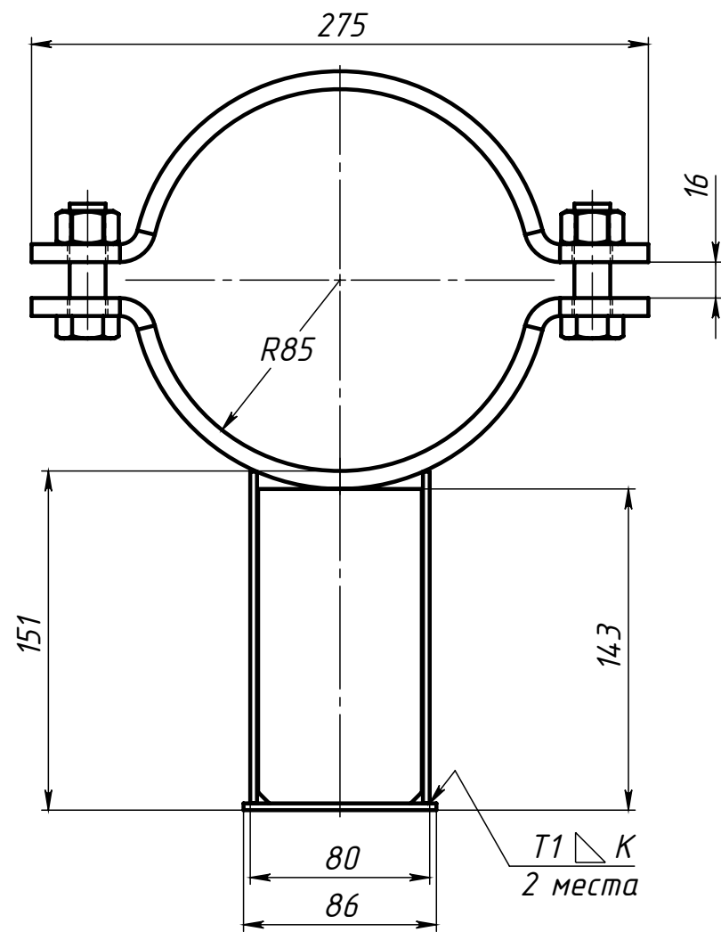
Поз.4 (Полухомут)
