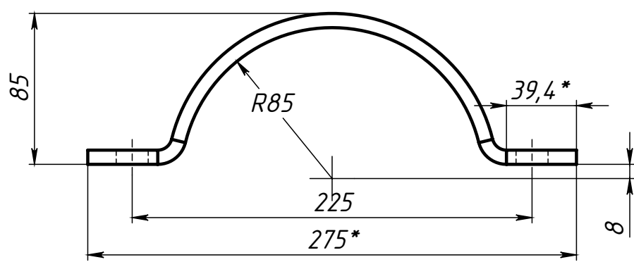
Поз.4 (Полухомут) развертка
